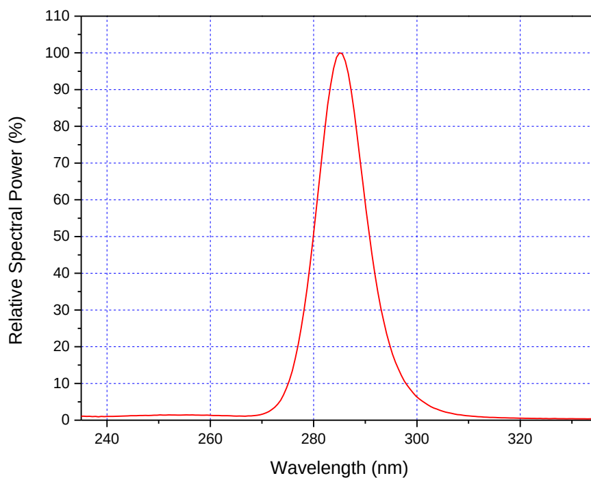
Fig 1. Spectrum, T_a=25^\circ\text{C} , I_F=20\text{mA}
